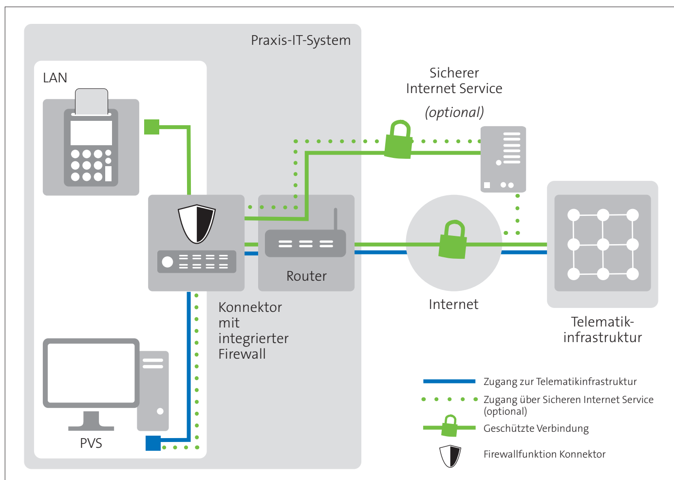
Grafik 2: Reihbetrieb mit Sicherem Internet Service
