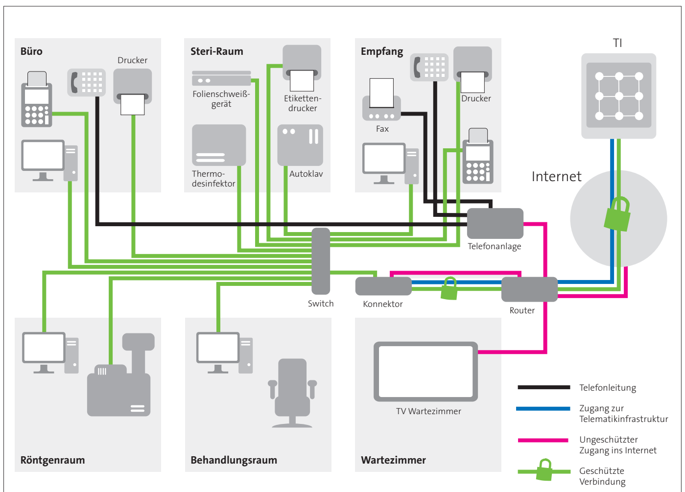
Grafik 1: Beispiel-Netzplan einer Praxis mit Reihenschaltung und Netztrennung
