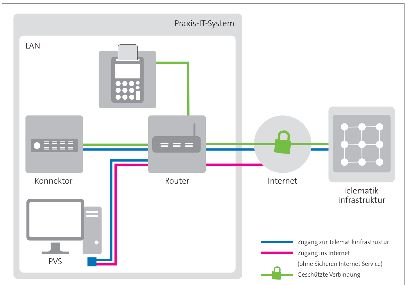
Grafik 3: Parallelbetrieb
